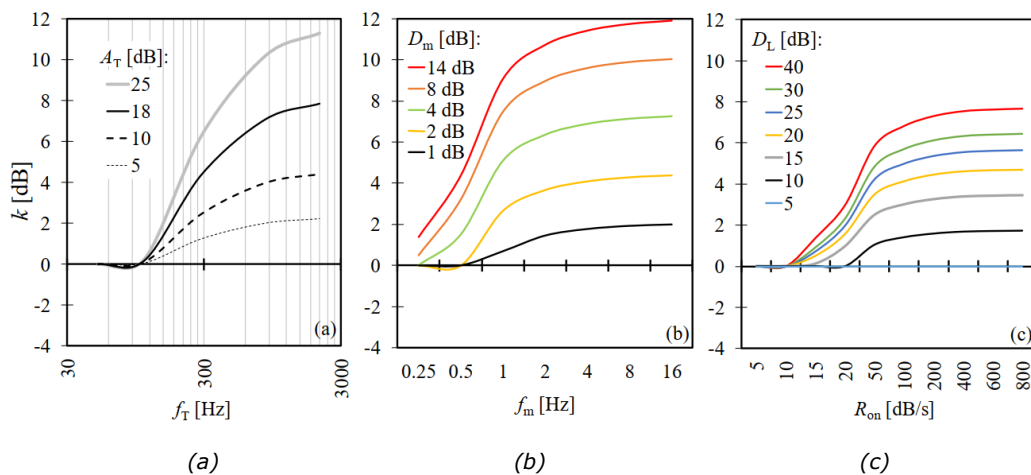
Kuva 4-1. (a) Kapeakaistamelun sanktion k riippuvuus ääneksen taajuudesta f_T ja ääneksen erottuvuudesta A_T . (b) Amplitudimoduloidun äänen sanktion riippuvuus modulaatiotaajuudesta f_m ja modulaatiosyvyydestä D_m . (c) Impulssimelun sanktion riippuvuus nousunopeudesta R_{on} ja taasoerosta DL (Keränen et al., 2019). Suomen lainsäädäntö ei kuitenkaan tunne sykinän sanktiomenettelyä.
