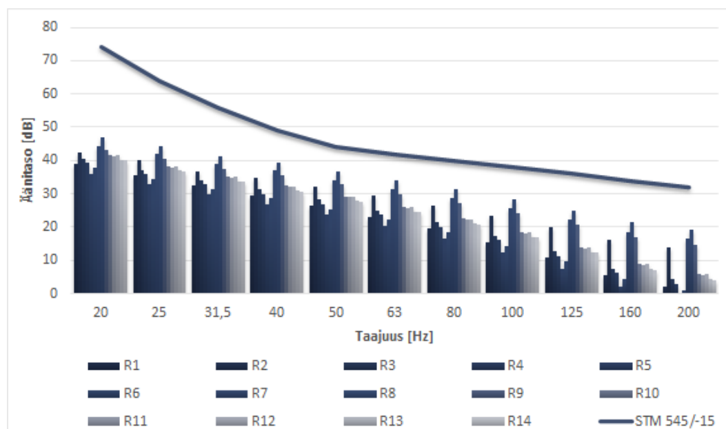
Kuva 3-2. Pientaajuisen melun laskentatulokset lähimmissä reseptoripisteissä R1-R14
